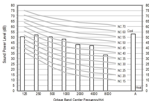
4) CNH364DB (AC036BN4DCH/AA)
