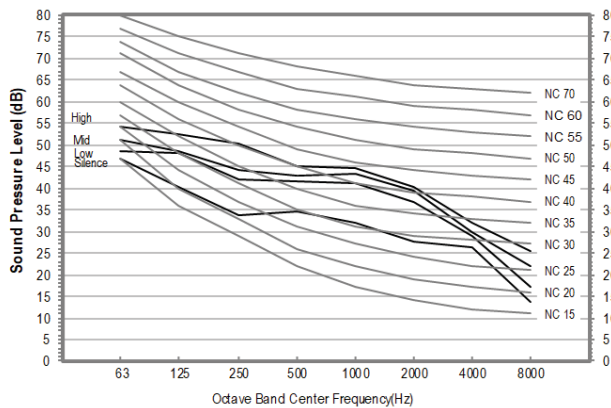
3) CNH30TDB (AC030BNTDCH/AA)
