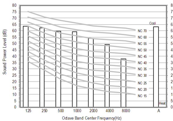
3) CNH30HDB (AC030BNHDCH/AA)
