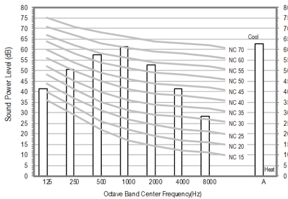
3) CNH30TDB (AC030BNTDCH/AA)
